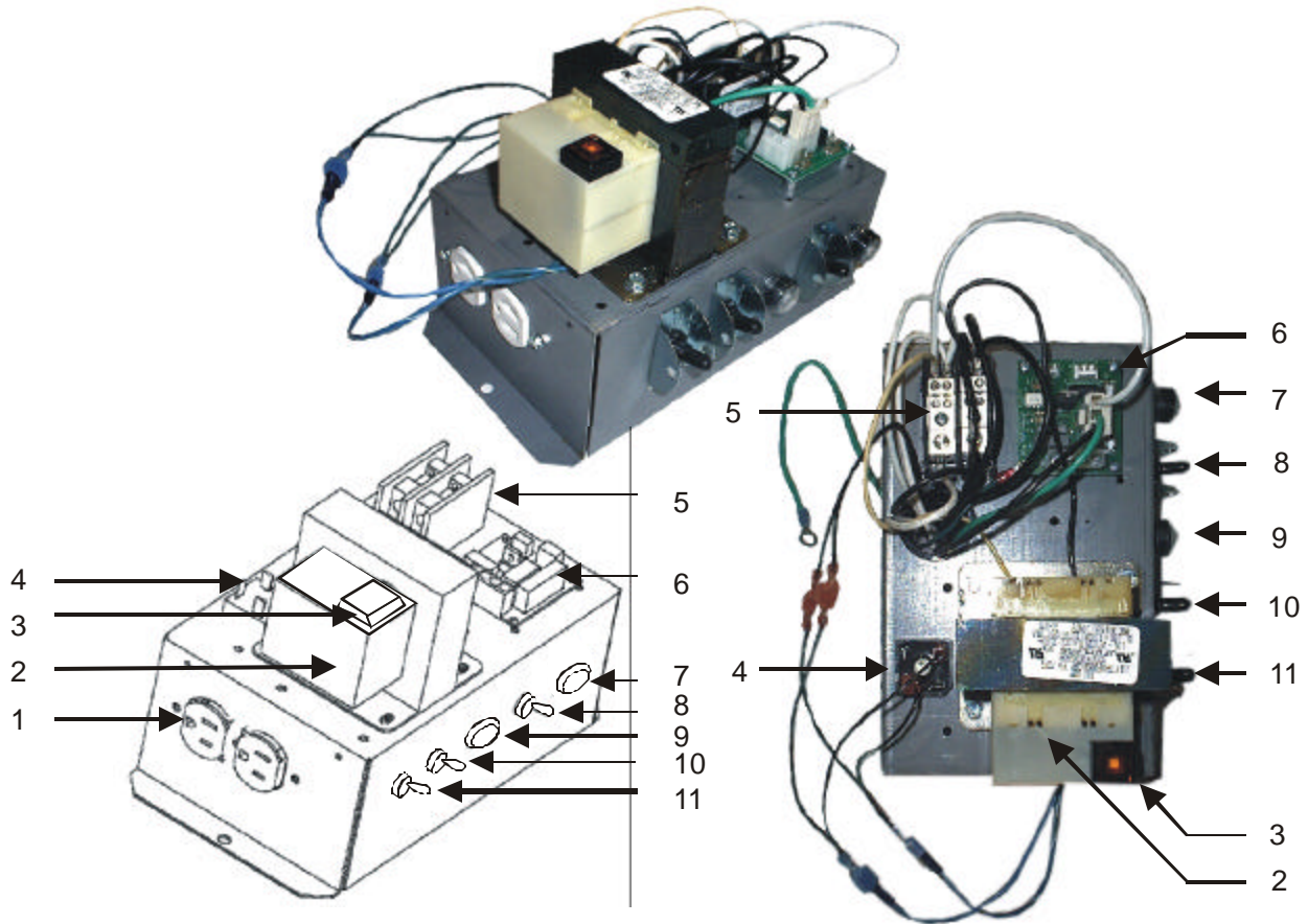
Fig. 7 (Power Box)
